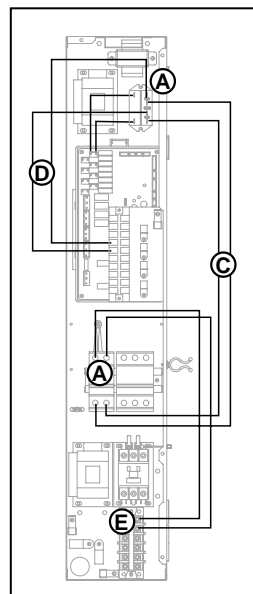
Résistance chauffante 3Ø
