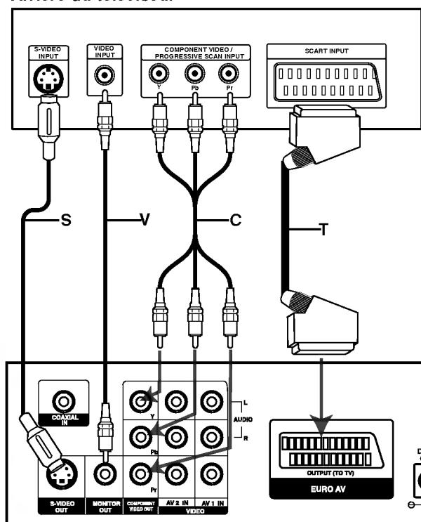
Panneau arrière du récepteur DVD
