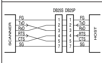
Fig. 2.01. RS232 options DB25
