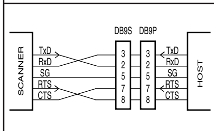
Fig. 2.02. RS232 options DB9
