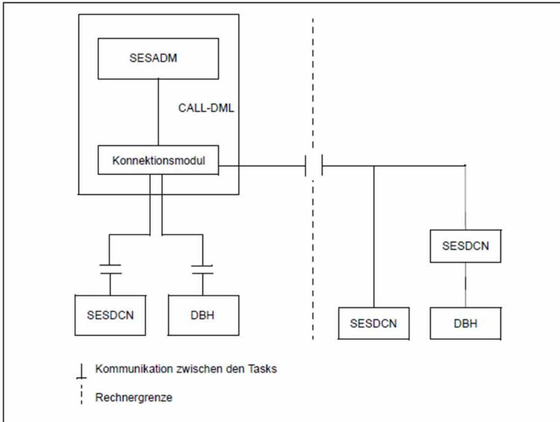
Bild 4: Administrationsschnittstelle SESADM
