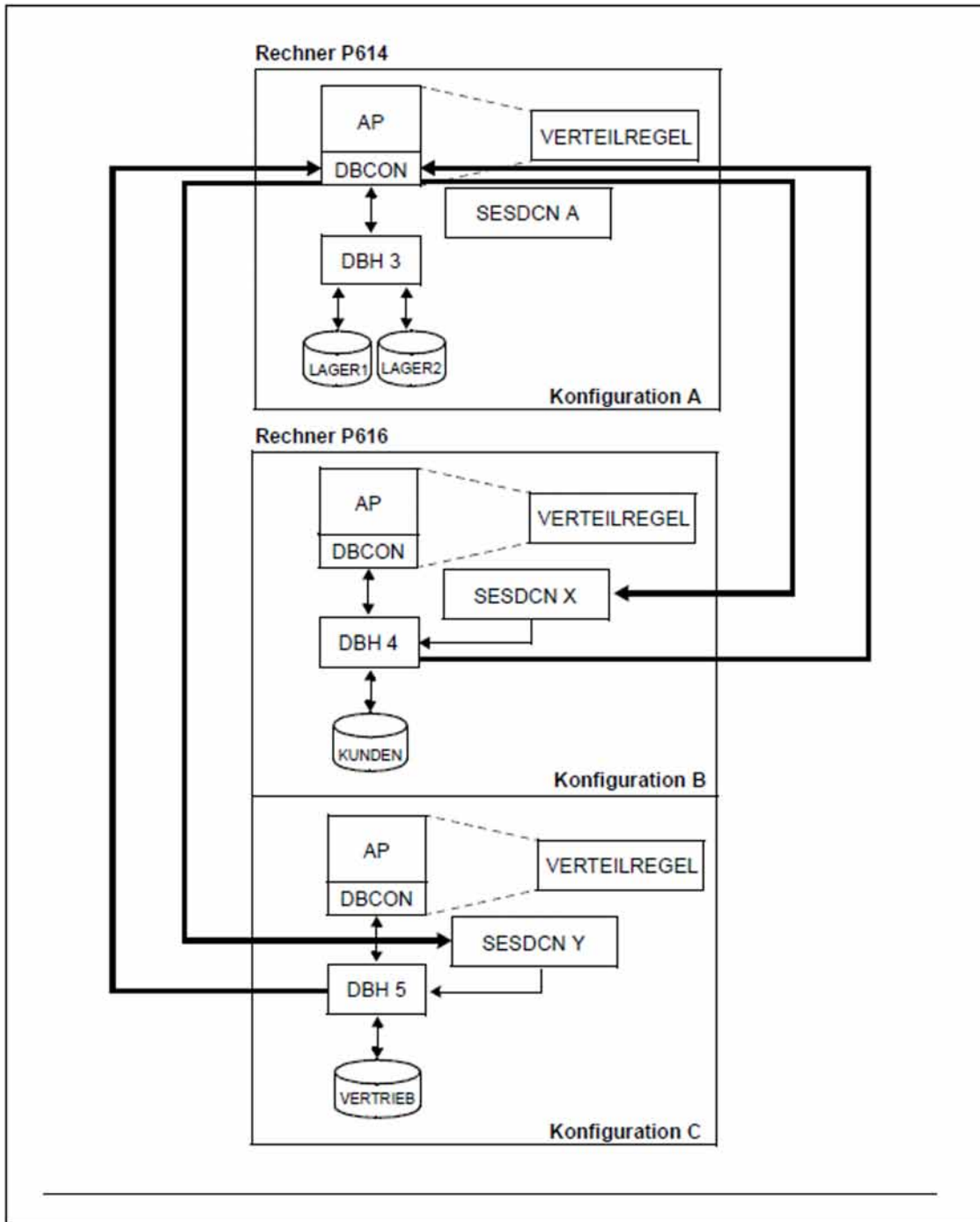
Bild 3: Beispiel für eine verteilte Anwendung mit remote Zugriff
