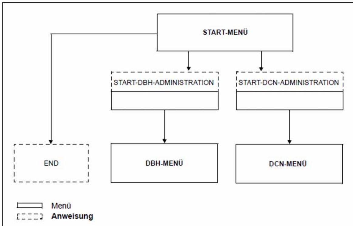
Bild 5: SDF-Auswahlmasken für die SESADM-Administration
