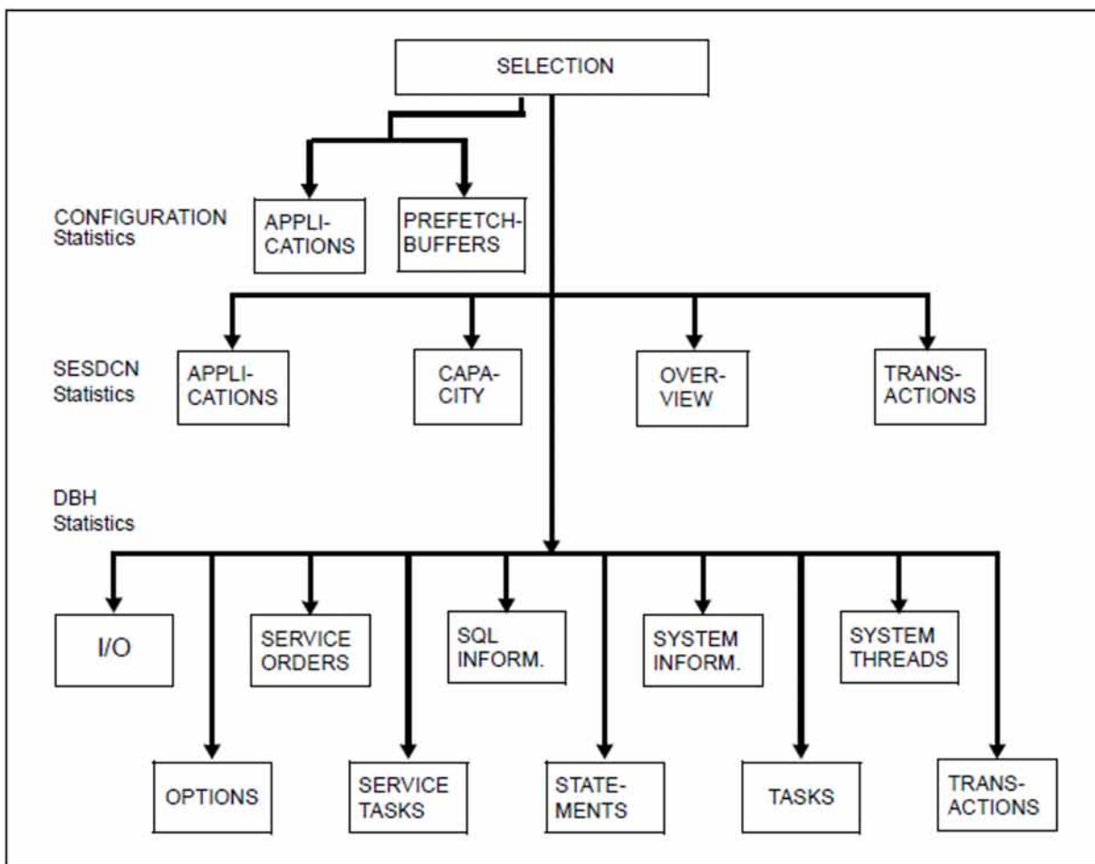
Bild 8: Statistikausgaben von SESMON
