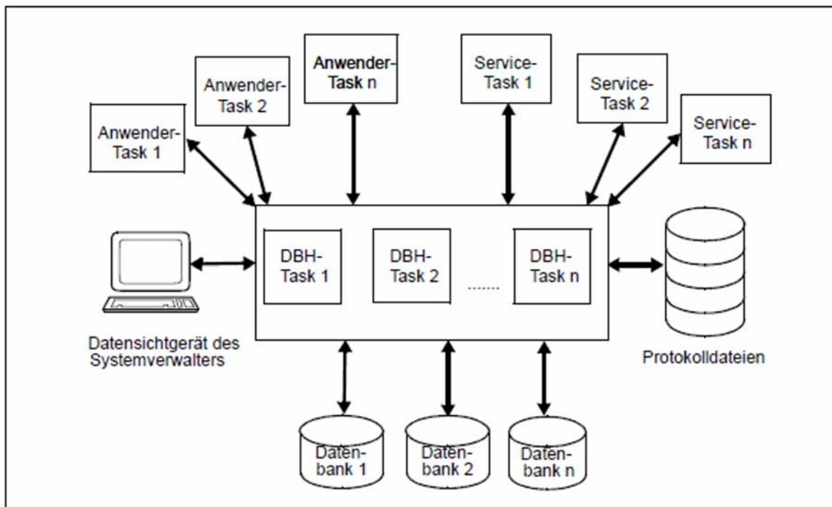
Bild 1: Aufgaben des SESAM/SQL-DBH
