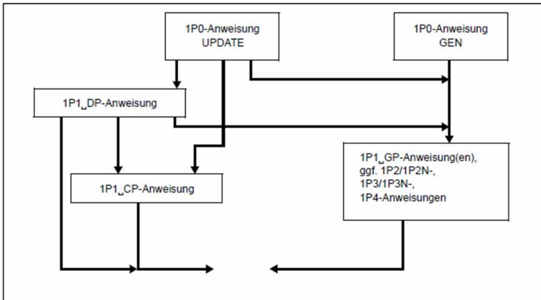
Bild 11: nach 1P0-Anweisung/Format 1 mögliche SEPA-Anweisungsfolgen
