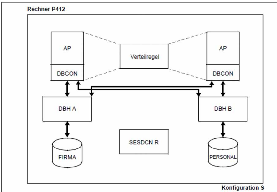
Bild 2: Beispiel für eine verteilte Anwendung mit lokalem Zugriff
