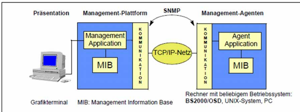
Bild 9: Kommunikation zwischen Management-Plattform und -Agenten über SNMP
