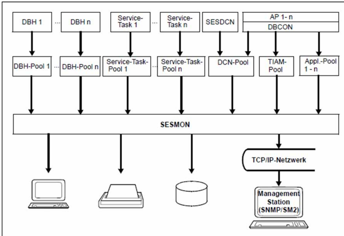
Bild 7: Sammlung und Auswertung der Daten mit SESMON
