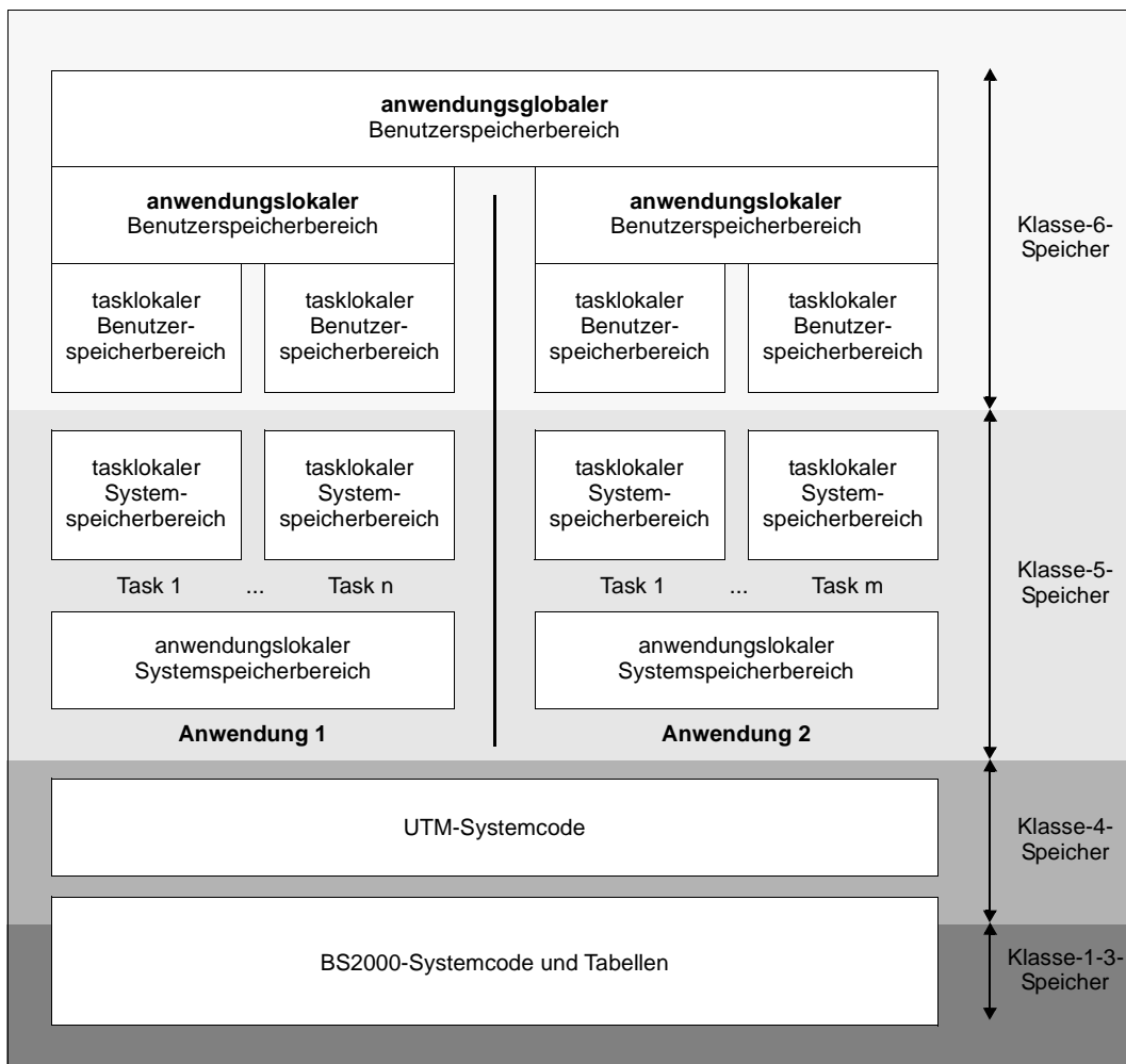
Bild 41: Speicherstruktur von UTM-Anwendungen auf BS2000-Systemen
