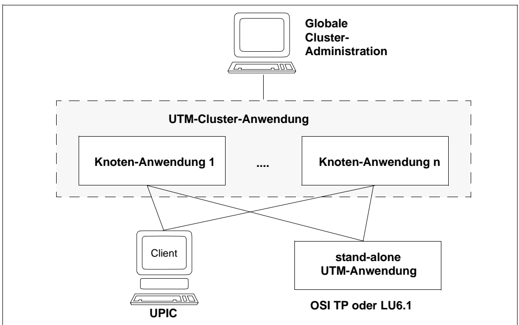
Bild 3: UTM-Cluster-Anwendung
