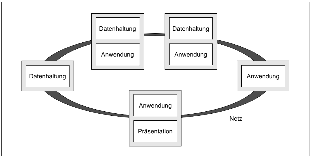
Bild 13: Multi-Tier-Architektur
