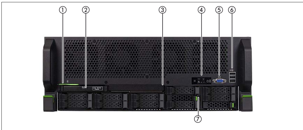
Bild 1: Server Unit (Frontseite)
