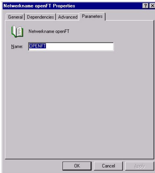
openFT im Cluster konfigurieren: Network Name - Parameters
