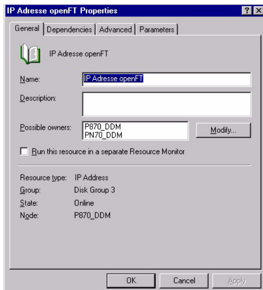
openFT im Cluster konfigurieren: IP Address - General
