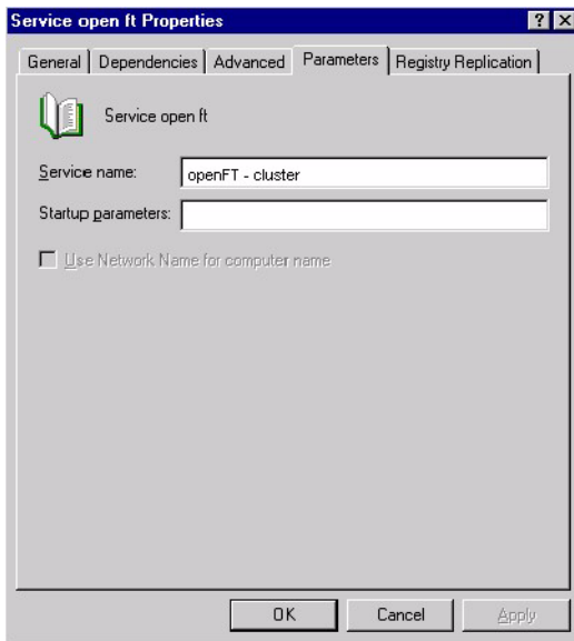
openFT im Cluster konfigurieren: Generic Service - Parameters
