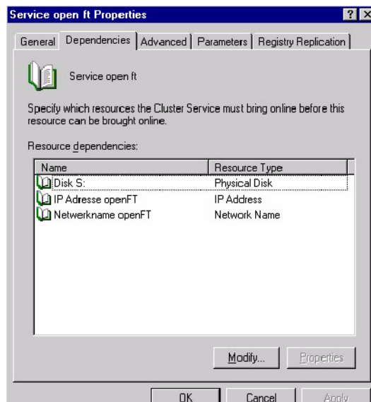
openFT im Cluster konfigurieren: Generic Service - Dependencies
