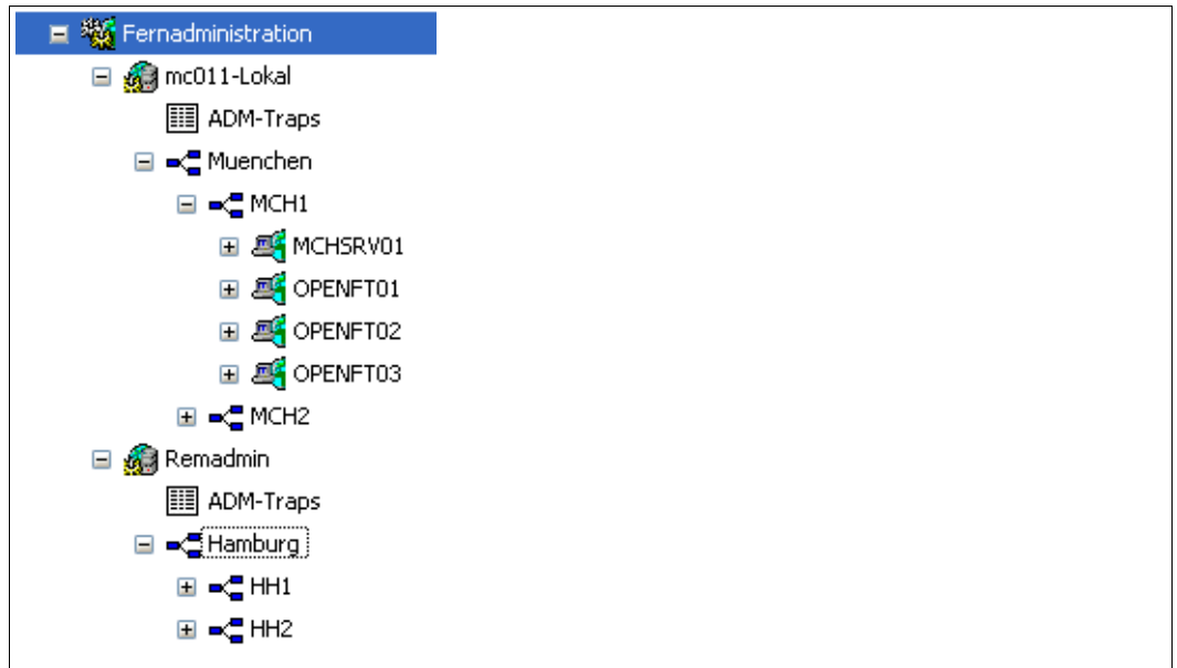
Lokaler und ferner Fernadministrations-Server im openFT Explorer
