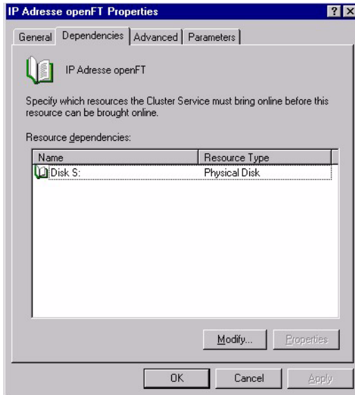
openFT im Cluster konfigurieren: IP Address - Dependencies
