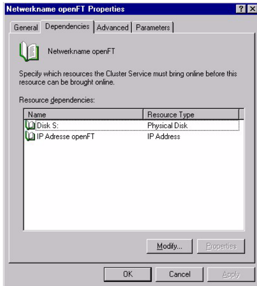
openFT im Cluster konfigurieren: Network Name - Dependencies
