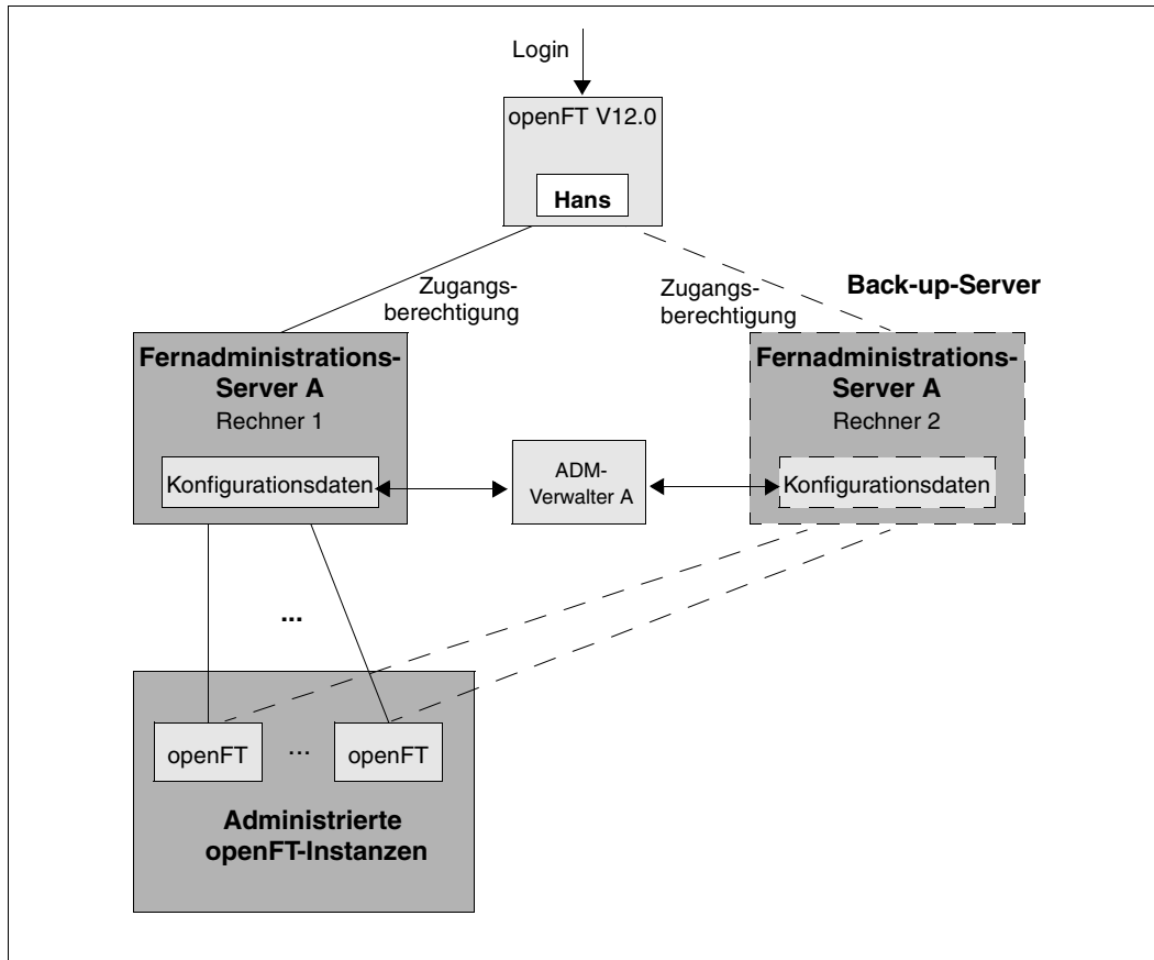
Redundante Konfiguration mit zweitem Fernadministrations-Server als Back-up
