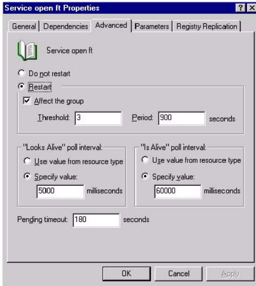
openFT im Cluster konfigurieren: Generic Service - Advanced
