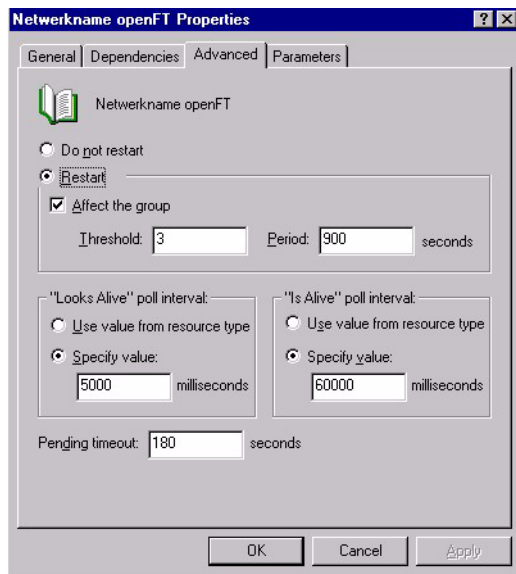
openFT im Cluster konfigurieren: Network Name - Advanced
