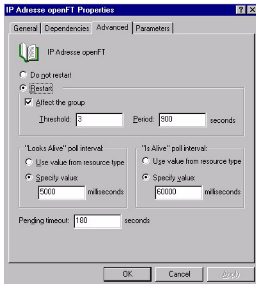
openFT im Cluster konfigurieren: IP Address - Advanced
