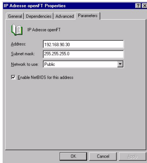
openFT im Cluster konfigurieren: IP Address - Parameters
