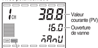
Avec potentiomètre
