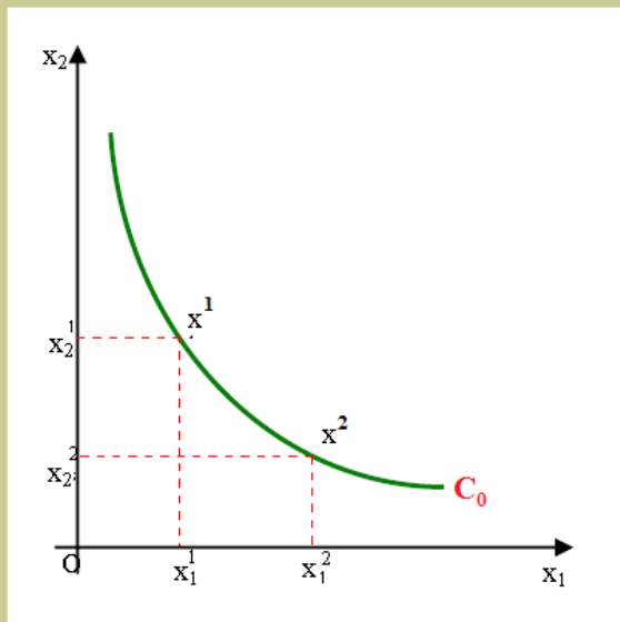
Figure 1.1 Courbe d'indifférence
