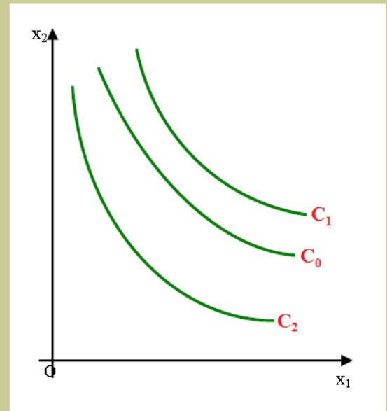
Figure 1.2 Carte d'indifférence
