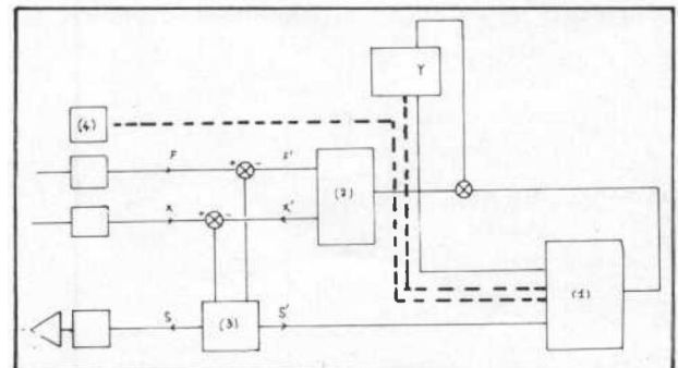
Figure 2 - (1) Calculateur programmé à partir du modèle et fournissant l'incrément \Delta t ; (2) (3) Opérateurs linéaires (4) Synchronisation.
