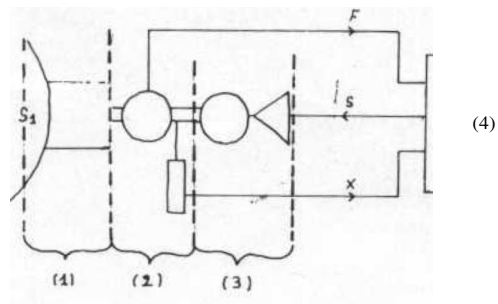
Figure 1 - Simulation d'un système mécanique lié au système 81 (1) Liaison (2) Capteurs (3) Moteurs (4) Calculateur (5) Transducteur.
