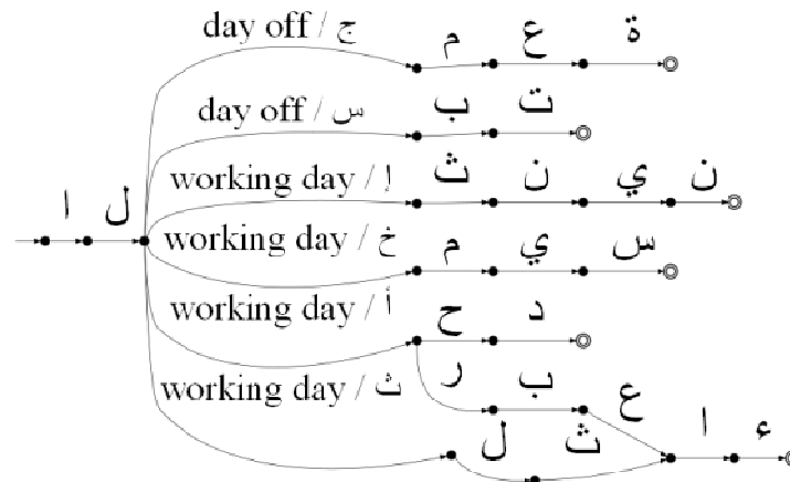
Figure 11 : Transducteur reconnaissant/stockant les sept jours de la semaine arabe et informant si le jour est ouvrable ou weekend en Algérie. Son automate sous-jacent est la déterminisation et minimisation de l'automate de la Figure 10.
