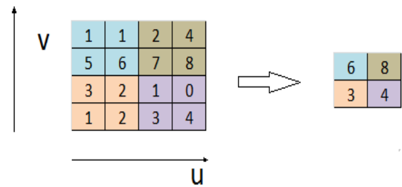
Fig. 3. Max pooling
