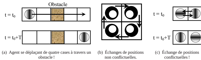
Figure 7. Quelques situations conflictuelles induites par les déplacements des agents [MAG 96].
