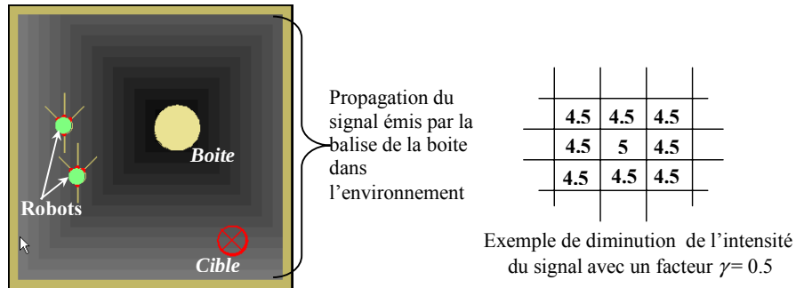
Figure 11. Émission de signaux à valeurs discrètes dans l'environnement
