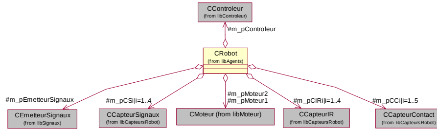
Figure 5. Schéma UML de l'organisation des classes d'un mini-robot ALICE simulé
