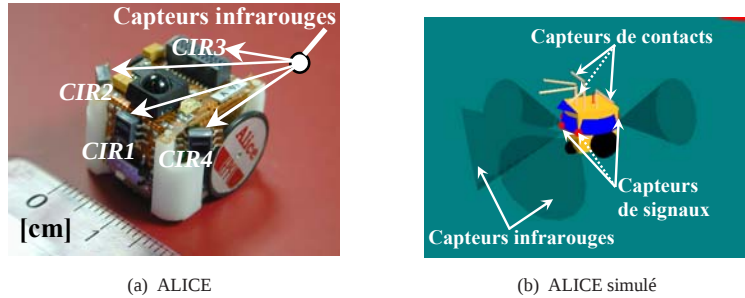
Figure 6. Modélisation du mini-robot ALICE
