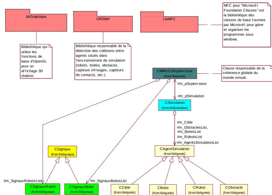
Figure 4. Schéma UML représentant les principales classes intervenant dans le cadre des simulations sous MiRoCo.
