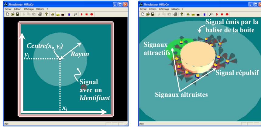
(a) Caractéristique d'un signal émis dans l'environnement.
