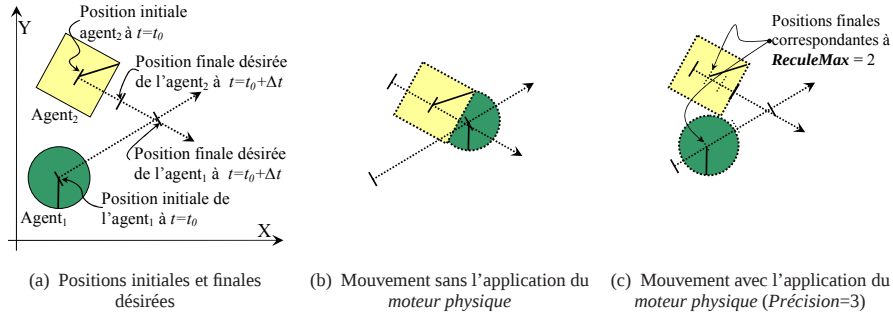
Figure 9. Application du moteur physique implémenté dans MiRoCo pour un cas simple de deux agents en mouvement.
