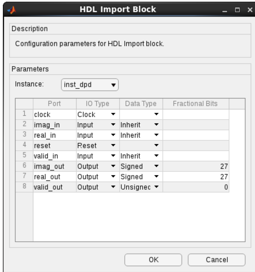
Figure 66. HDL Import inst_dpd Parameters
