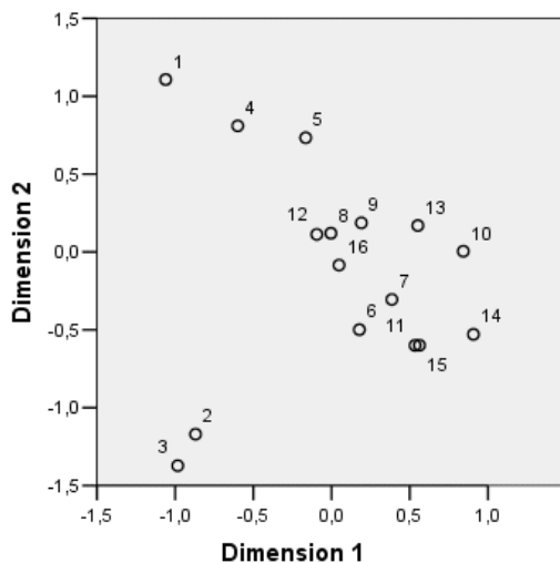
Figure 10-39 Points de modalité de l'interaction moment/diagnostic
