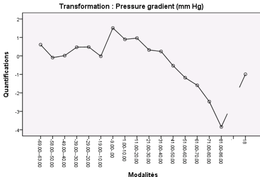
Figure 9-33 Diagramme de transformation de la variable Gradient de pression (nominal)
