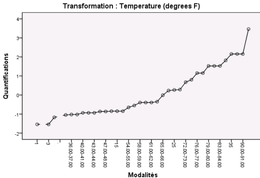
Figure 9-42 Diagramme de transformation de la variable Température (ordinal)
