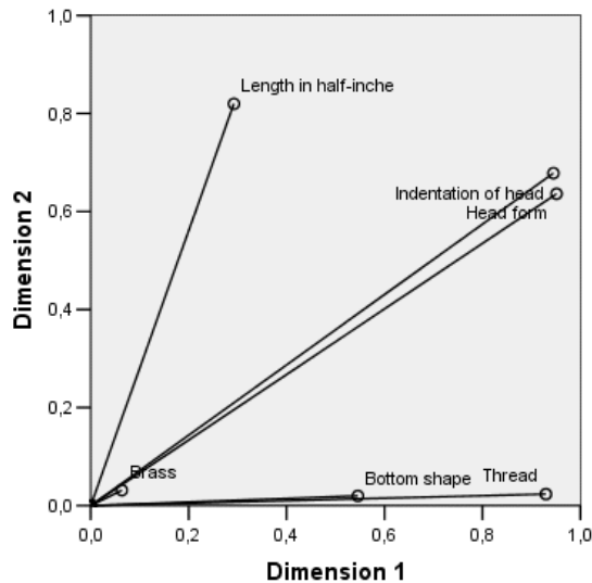
Figure 13-7 Diagramme des mesures de discrimination
