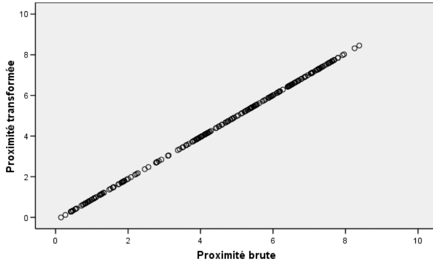
Figure 15-30 Diagramme de transformation
