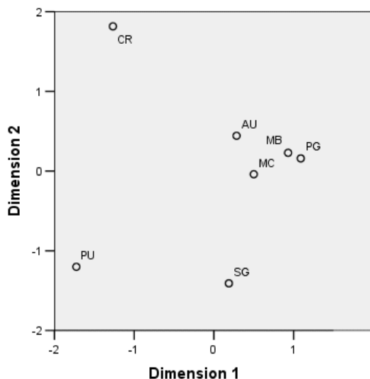
Figure 10-12 Diagramme des coordonnées principales
