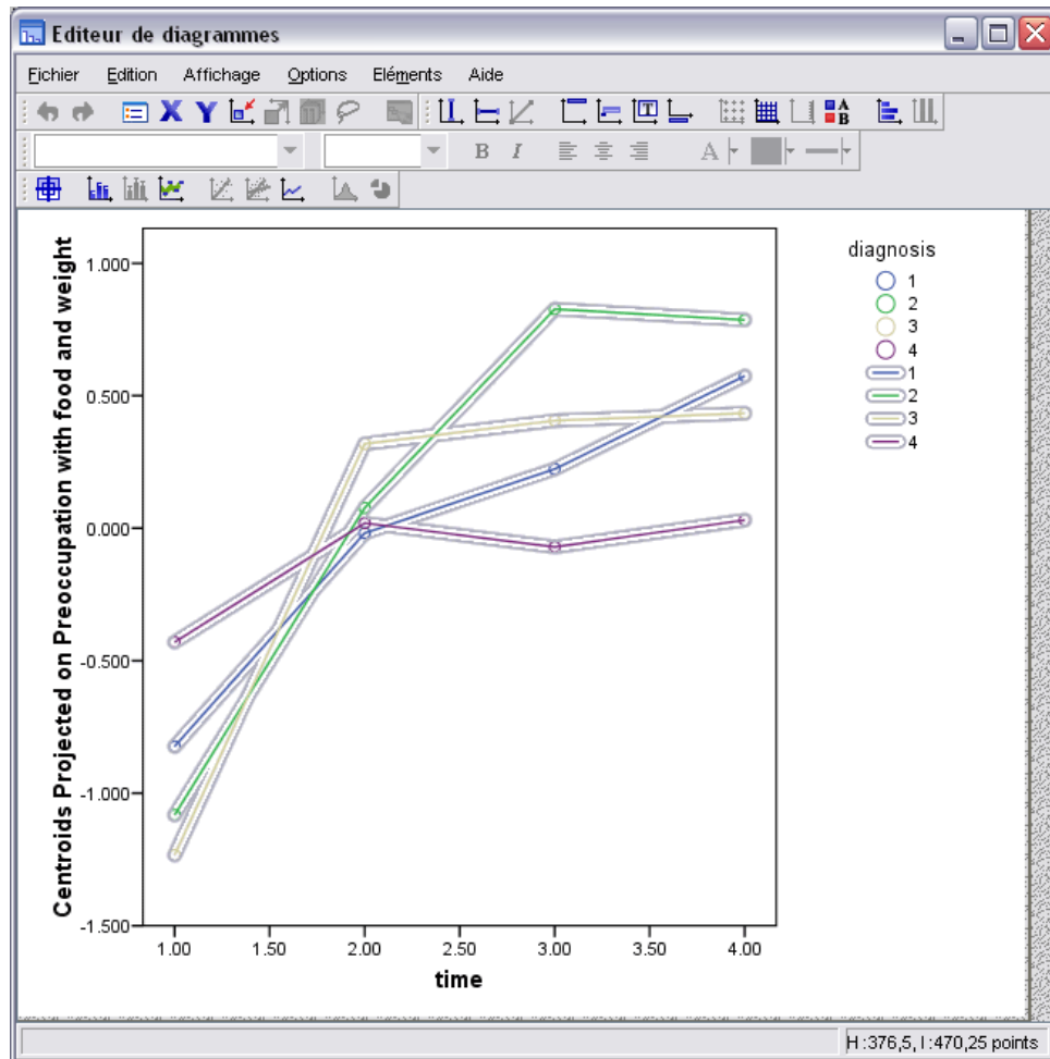
Figure 10-54 Projection dans le temps des barycentres des moments de diagnostic sur la préoccupation du corps
