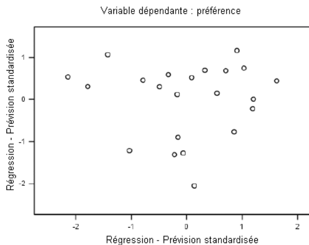
Figure 9-6 Résidus et prévisions
