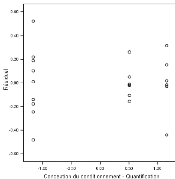
Figure 9-24 Résidus de la régression nominale
