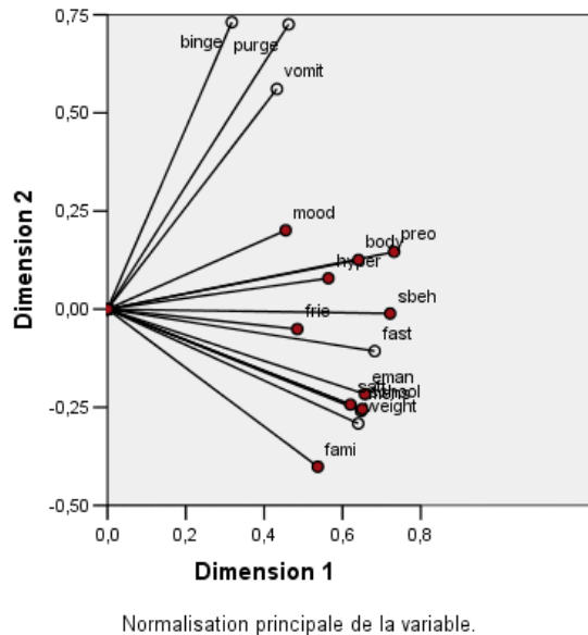
Figure 10-36 Diagramme des corrélations entre composantes
