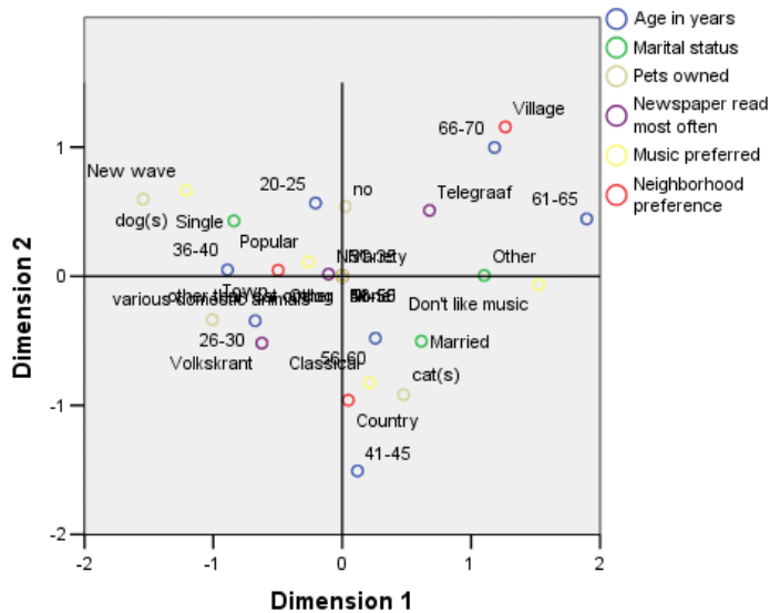
Figure 11-32 Barycentres étiquetés par des variables (âge, nominal)
