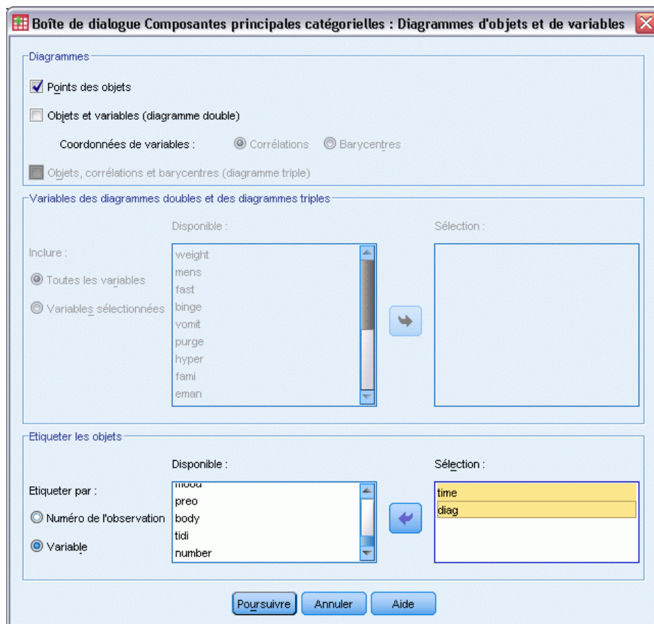
Figure 3-9 Diagrammes d'objets et de variables
