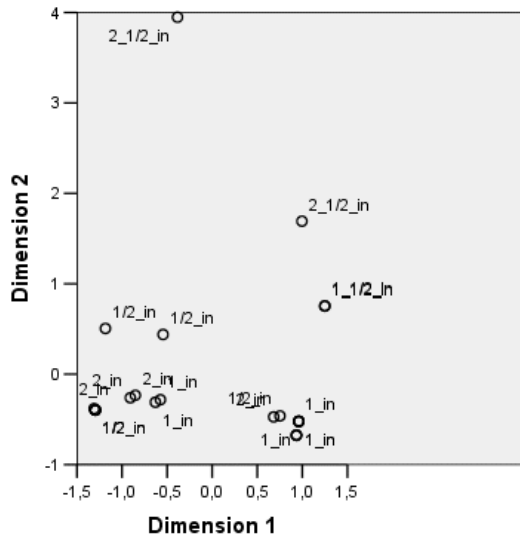
Figure 13-11 Coordonnées des objets étiquetées avec Longueur en demi-pouces
