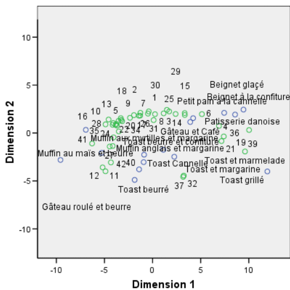
Figure 15-16 Diagramme joint de l'espace individuel Petit-déjeuner avec jus de fruit, jambon, oeufs et boisson
