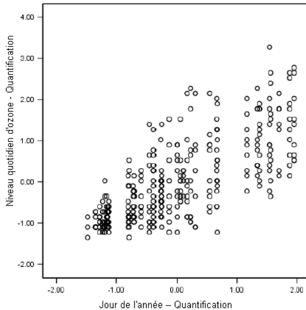
Figure 9-57 Diagramme de dispersion des variables transformées
