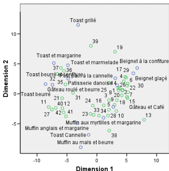
Figure 15-7 Diagramme joint de l'espace commun pour une solution non dégénérée
