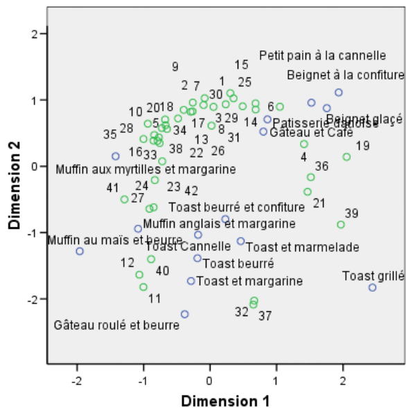
Figure 15-13 Diagramme joint de l'espace commun
