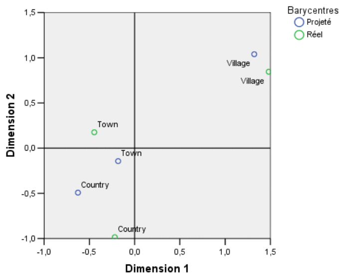
Figure 11-25 Barycentres et barycentres projetés de Préférence de voisinage
