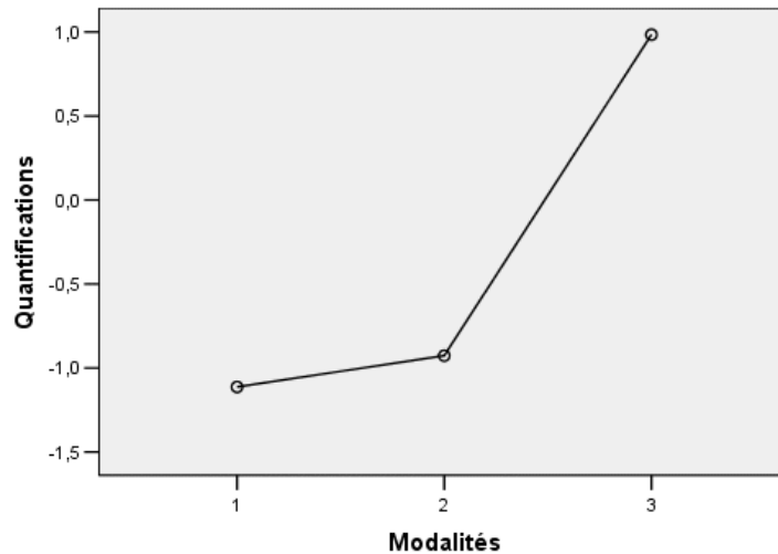
Figure 10-33 Diagramme de transformation des antécédents scolaires/professionnels
