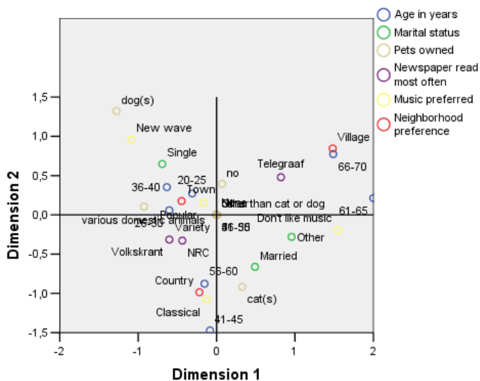
Figure 11-22 Barycentres étiquetés par des variables
