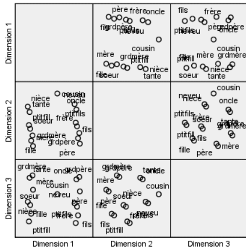
Figure 14-20 Coordonnées de l'espace commun
