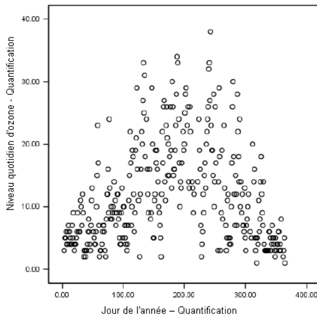
Figure 9-48 Diagramme de dispersion du niveau d'ozone quotidien par jour de l'année
