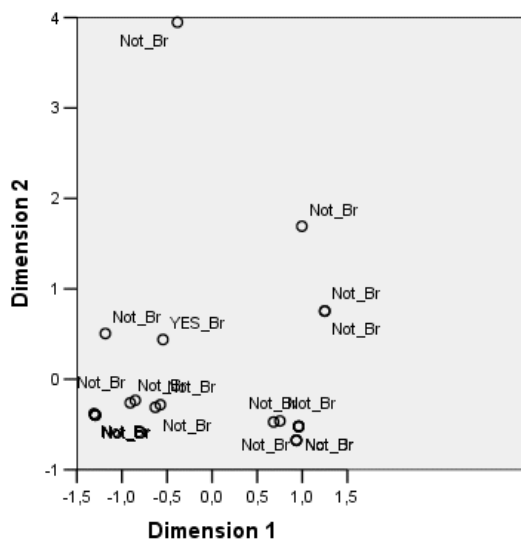
Figure 13-12 Coordonnées des objets étiquetées avec la variable Cuivre
