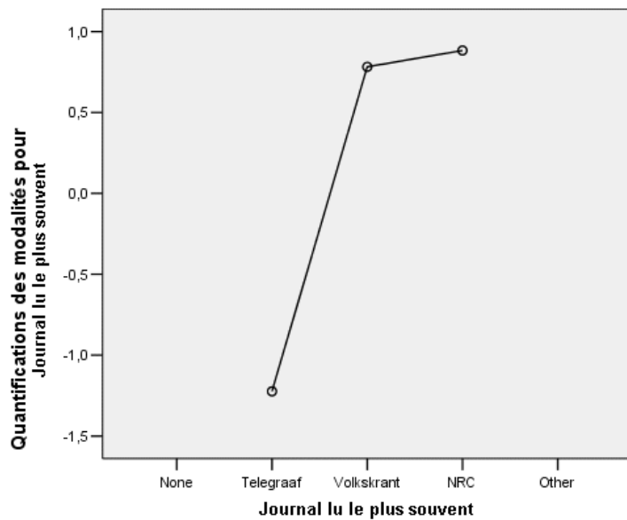
Figure 11-19 Diagramme de transformation de la variable Journal lu le plus souvent (nominale)
