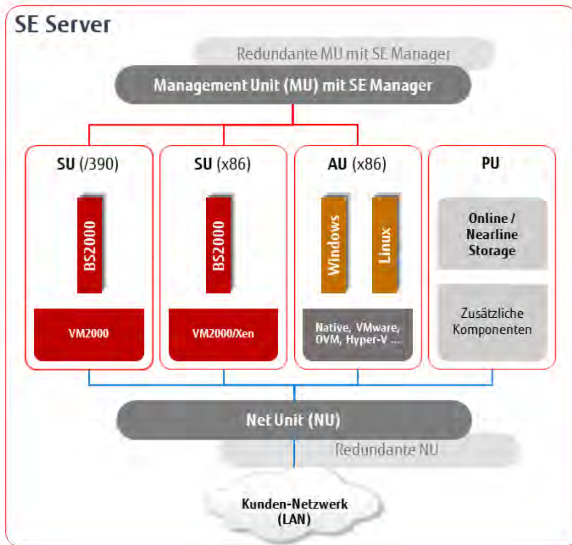
Bild 1: Architektur der SE Server
