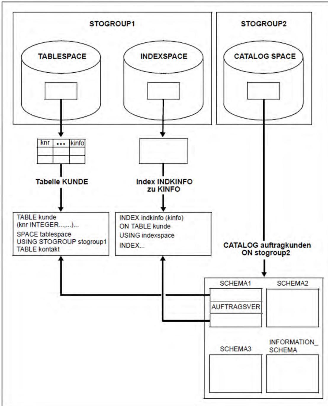
Bild 7: Beispiel einer SESAM/SQL-Datenbank
