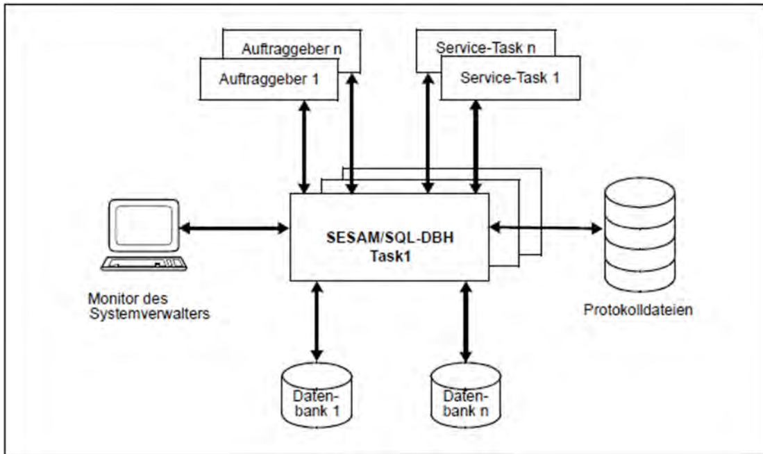
Bild 25: Der SESAM/SQL-DBH und seine Schnittstellen
