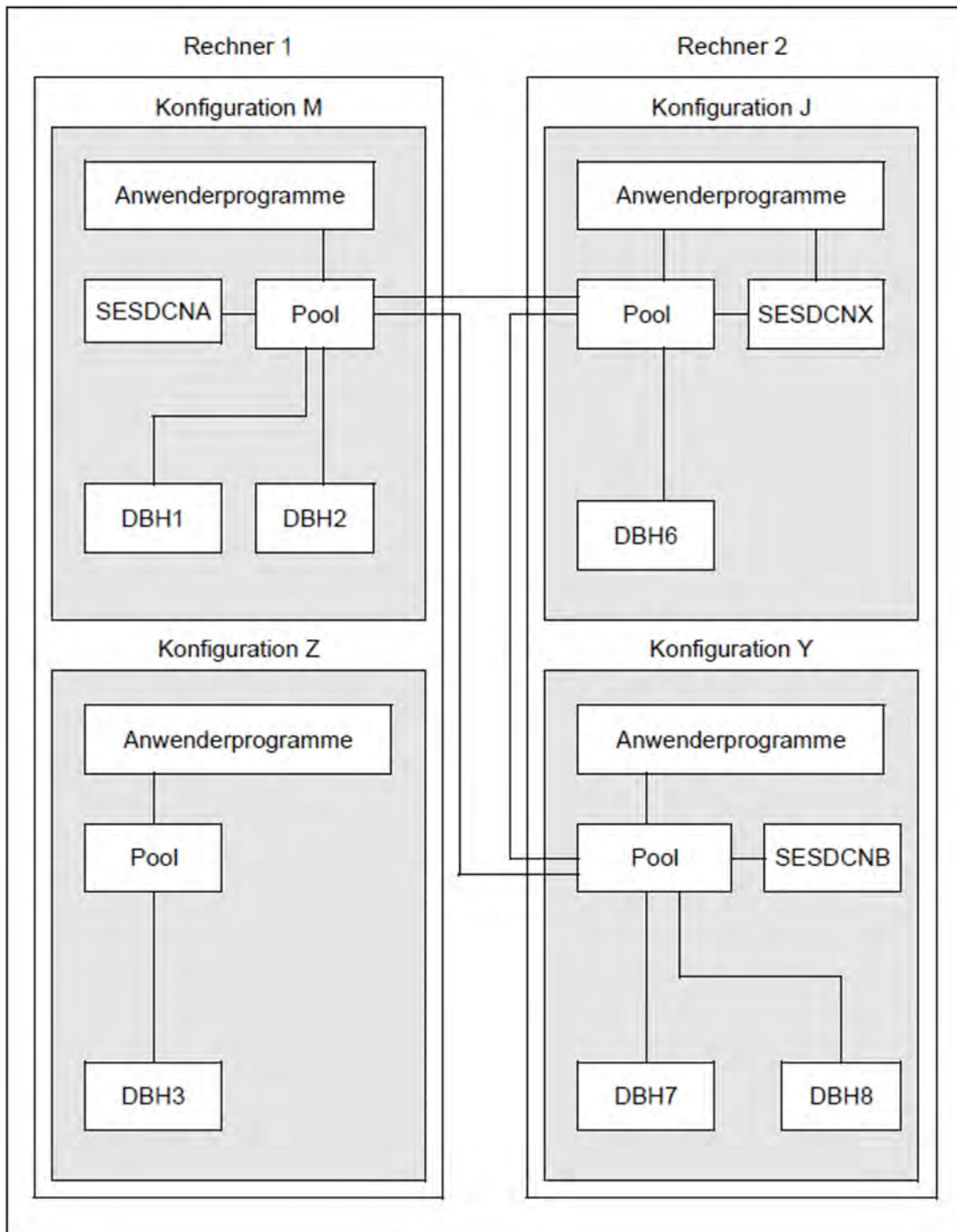
Bild 27: Beispiel für die Kommunikation zwischen Konfigurationen
