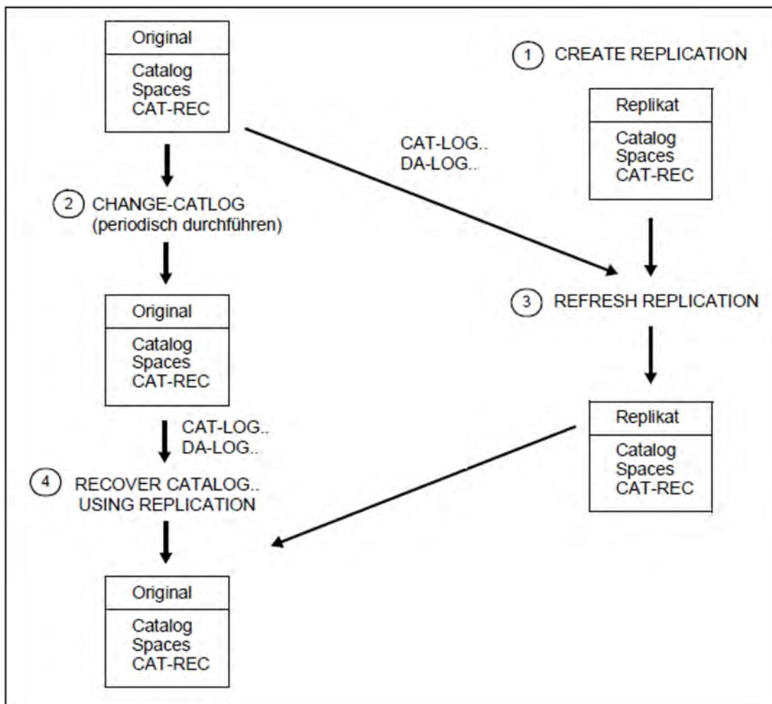
Bild 23: Nutzung eines Replikats als Schattendatenbank
