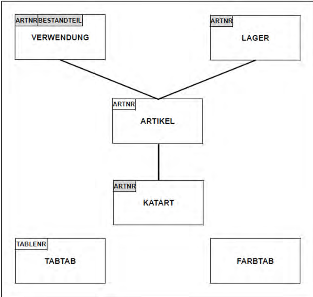
Bild 6: Basistabellen des Schemas TEILE; referenzierende Fremdschlüssel sind grau unterlegt
