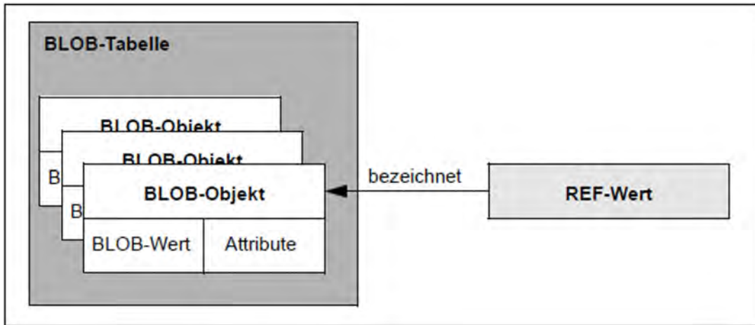
Bild 8: Struktur der BLOB-Konstrukte
