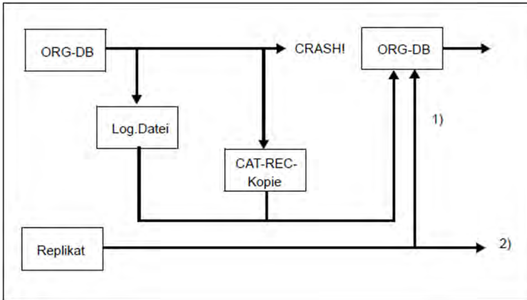
Bild 22: Originaldatenbank mit Hilfe eines Replikats reparieren
