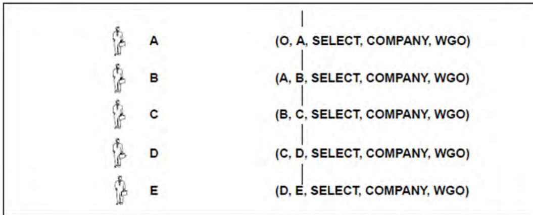
Bild 10: Weitergabe eines Privilegs
