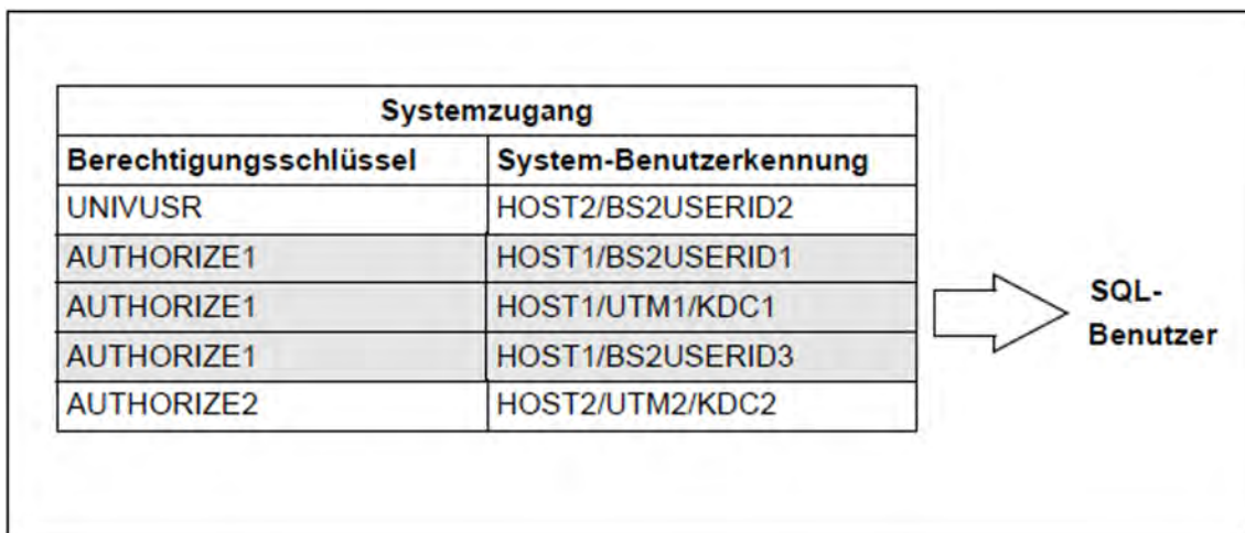
Bild 35: Beispiel für Systemzugänge eines SQL-Benutzers
