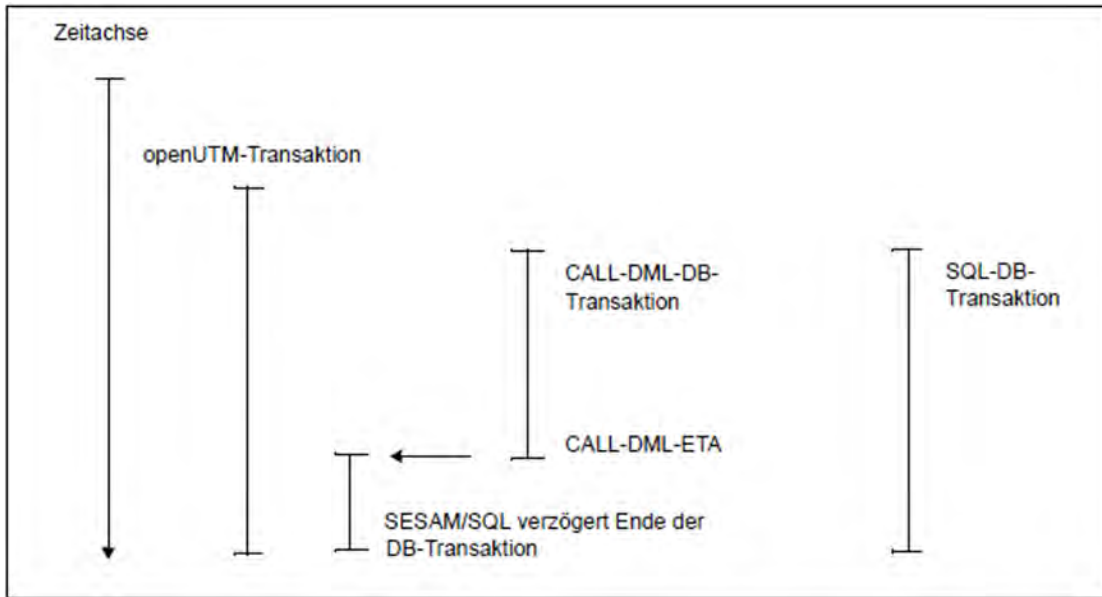
Bild 36: Synchronisation von DB-Transaktion und openUTM-Transaktion
