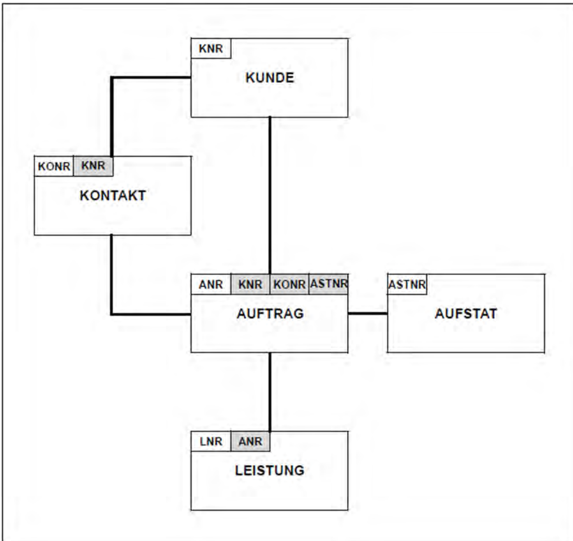
Bild 5: Basistabellen des Schemas AUFTRAGSVER; referenzierende Fremdschlüssel sind grau unterlegt
