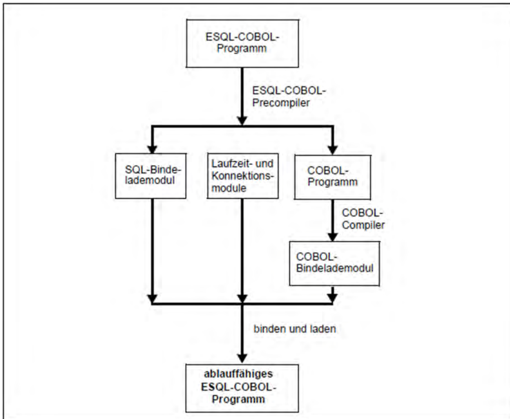
Bild 3: Einsatz des ESQL-Precompilers
