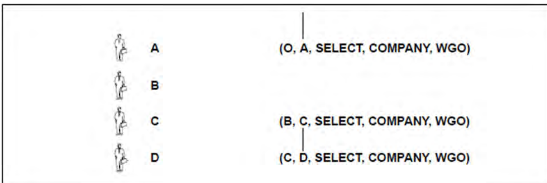
Bild 12: Hypothetische Situation: abgetrennte Privilegien
