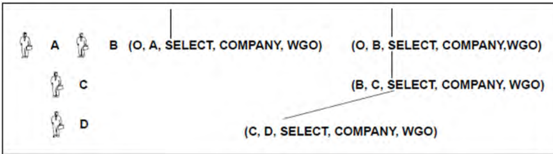
Bild 14: Entzug des Privilegs (A, C, SELECT, COMPANY, WGO)
