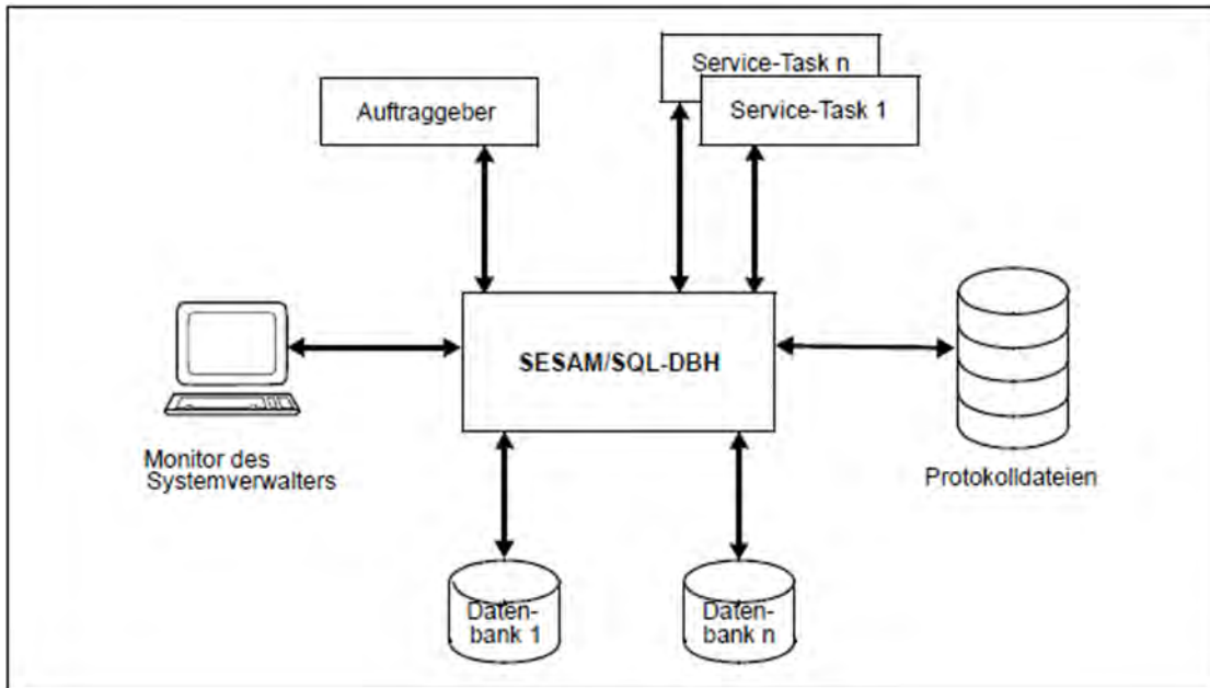
Bild 26: Der SESAM/SQL-LINK-DBH und seine Schnittstellen
