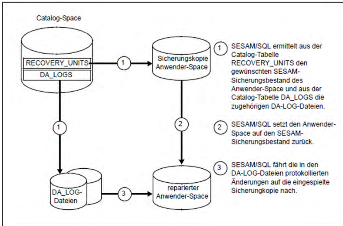
Bild 19: Reparatur eines Anwender-Space
