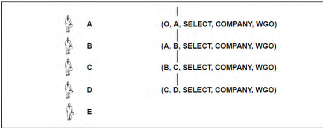
Bild 11: Entzug des Privilegs (D,E,SELECT,COMPANY,WGO)
