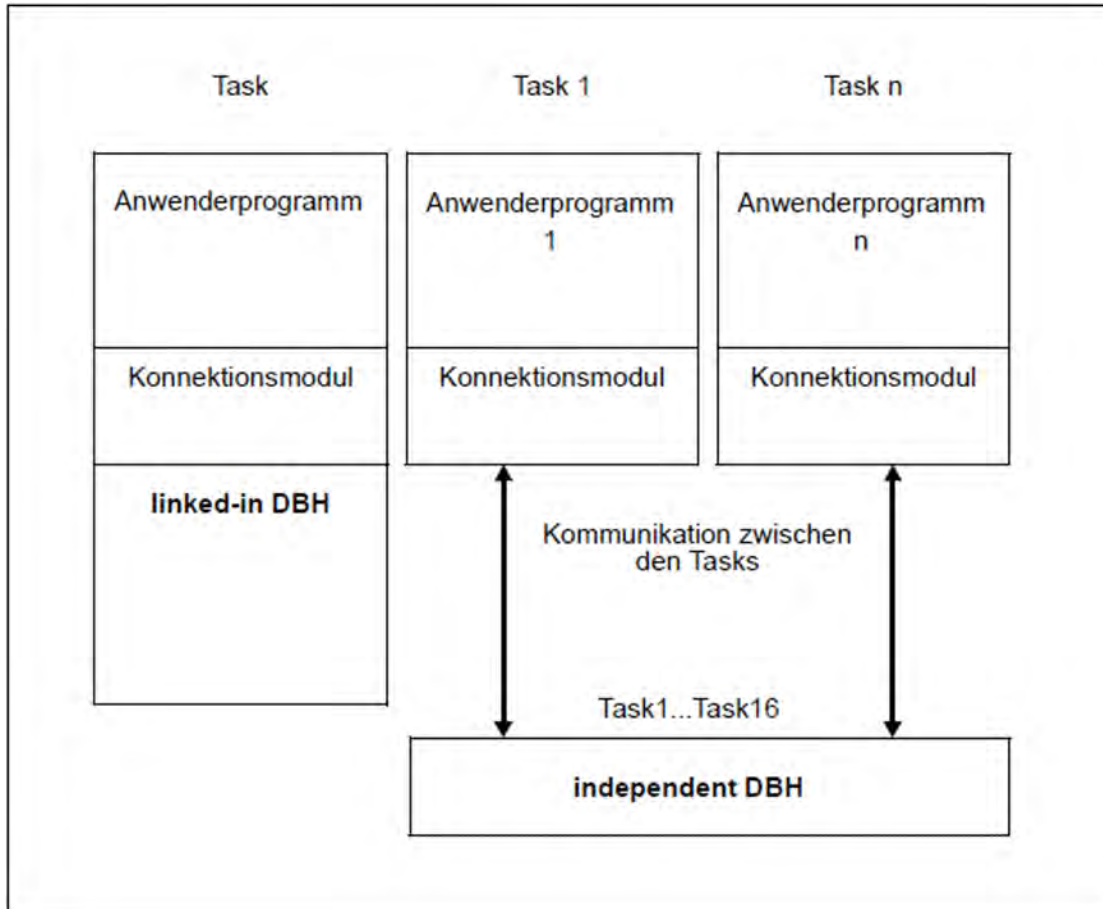
Bild 24: Gegenüberstellung von linked-in DBH und independent DBH
