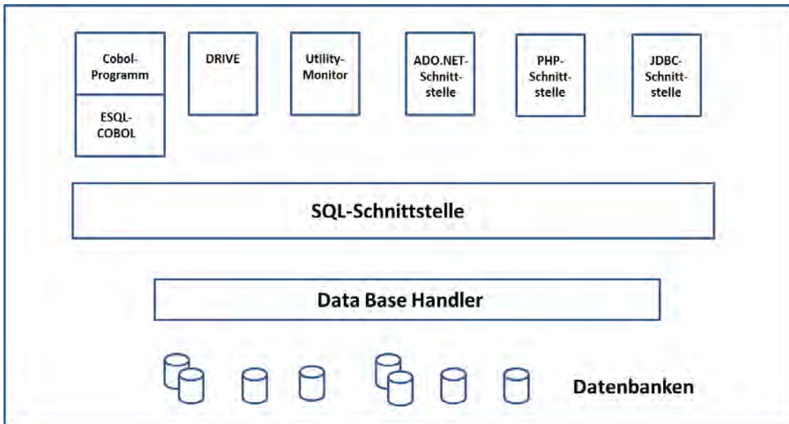
Bild 1: SQL-Schnittstelle
