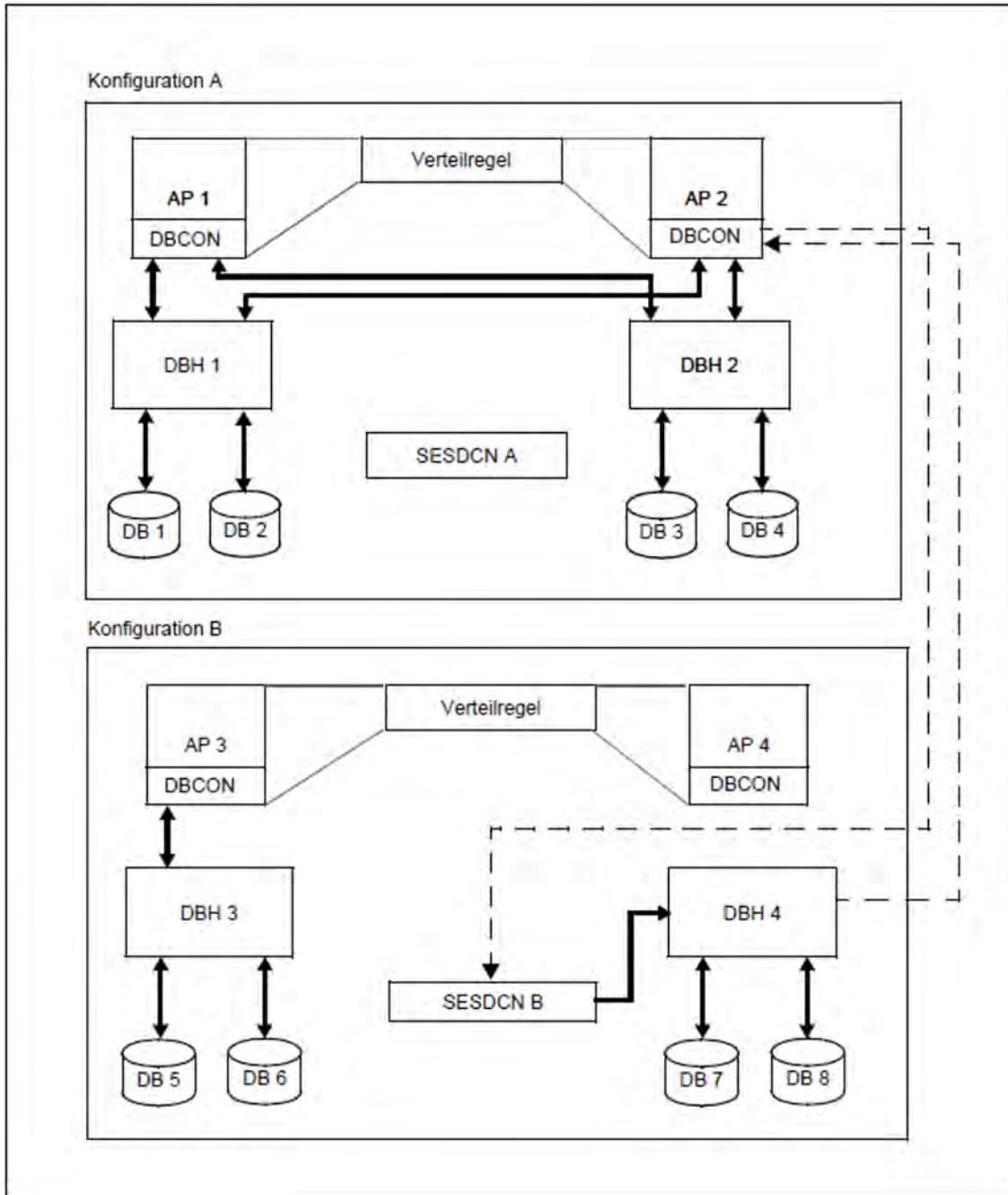
Bild 28: Verteilte Verarbeitung
