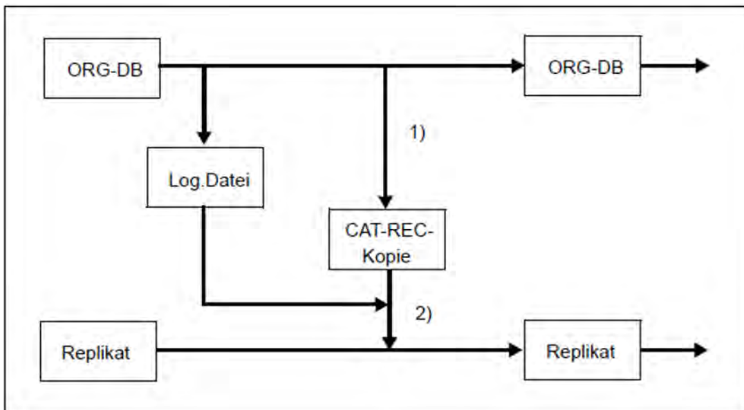
Bild 21: Replikat aktualisieren
