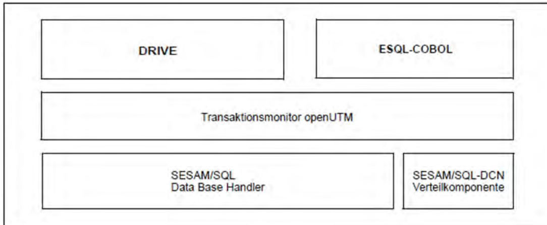
Bild 2: Entwicklungswerkzeuge
