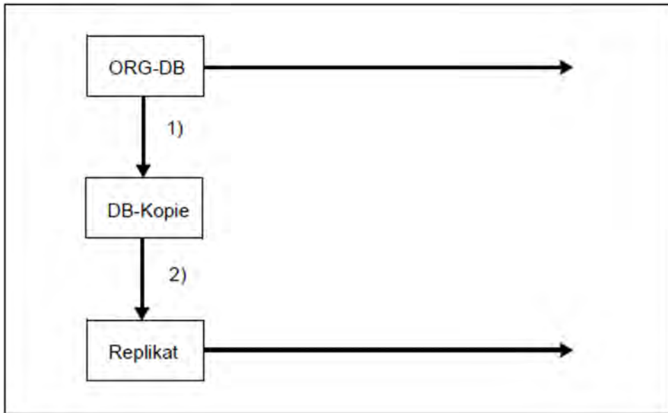
Bild 20: Replikat erstellen
