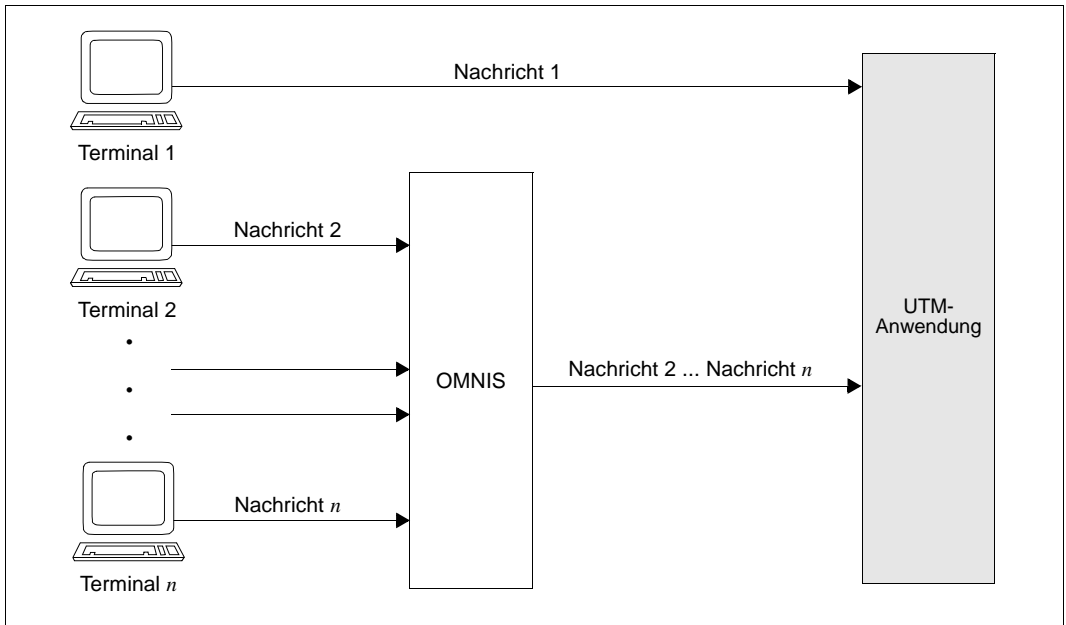
Bild 17: Kombination von Multiplex- und direkten Verbindungen
