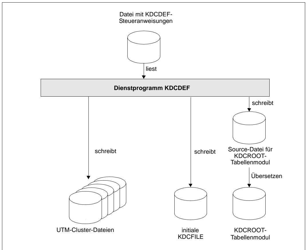
Bild 5: Ergebnis des KDCDEF-Laufs (bei OPTION ...,GEN=(KDCFILE, ROOTSRC, CLUSTER)) für eine UTM-Cluster-Anwendung
