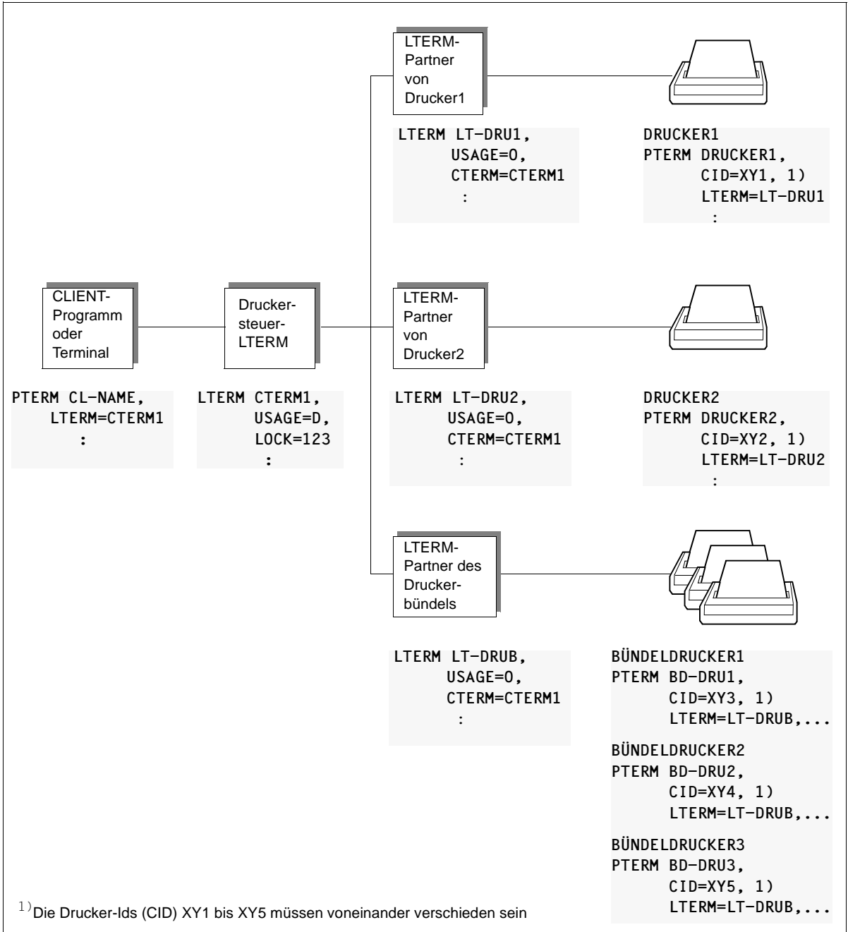
Bild 14: Konfiguration eines Druckersteuer-LTERMs und der zugehörigen Drucker
