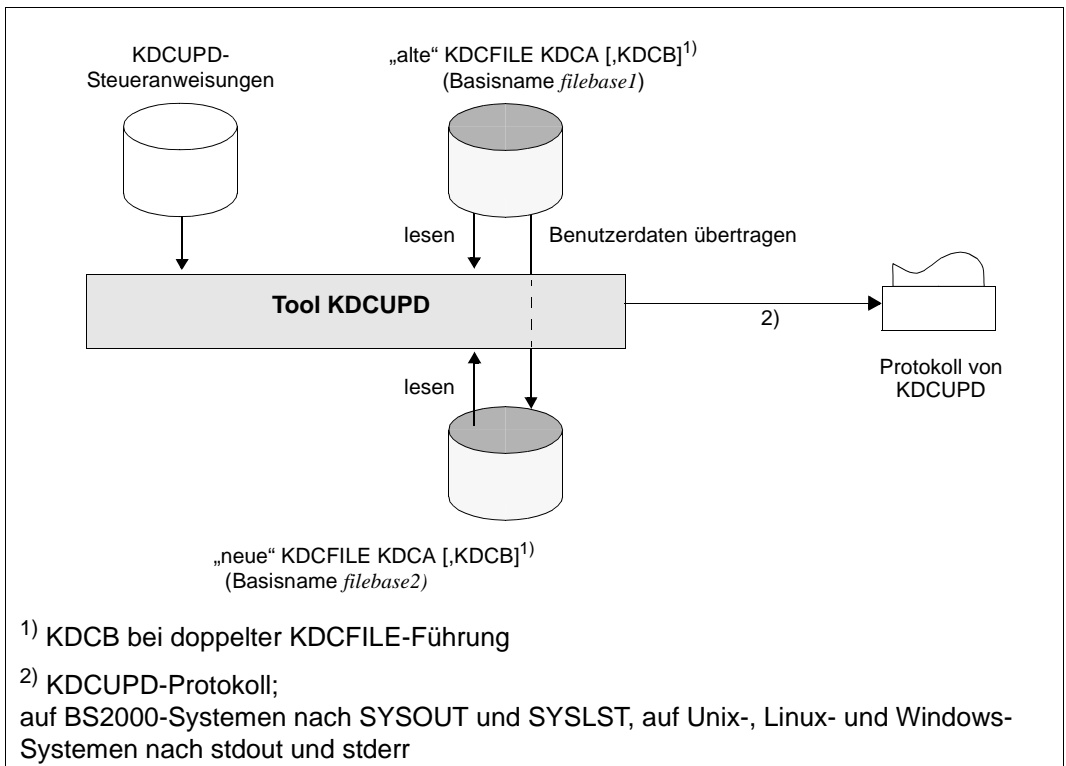
Bild 20: KDCFILE aktualisieren
