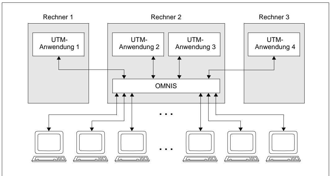
Bild 15: Nachrichtenverteilung und Multiplexing mit OMNIS
