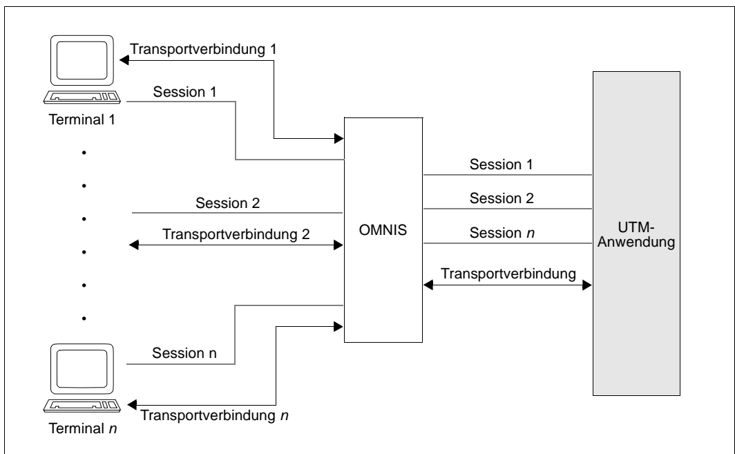
Bild 16: Transportverbindungen und Sessions beim Multiplexen
