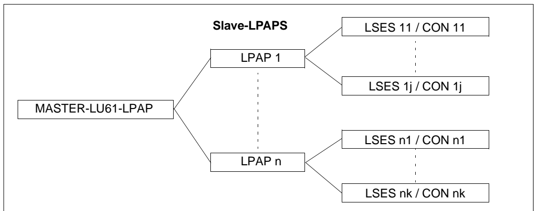
Bild 7: Beispiel LU6.1-LPAP-Bündel
