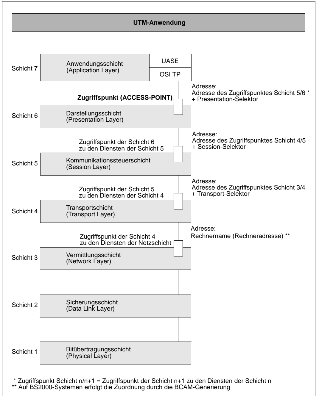
Bild 8: Adressen der Dienstzugriffspunkte im OSI-Referenzmodell
