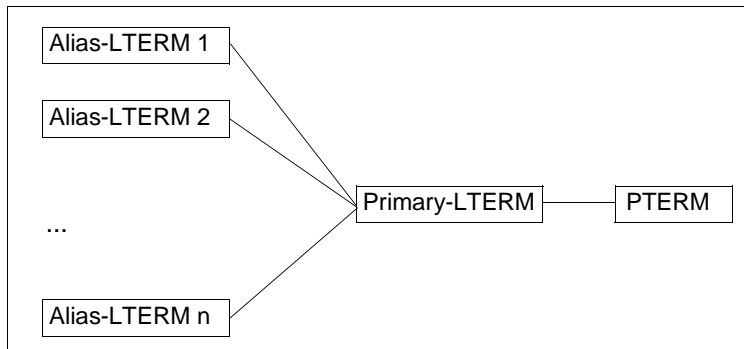
Bild 12: Beispiel LTERM-Gruppe
