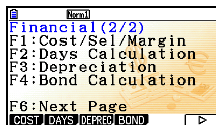
Écran Finance 2
