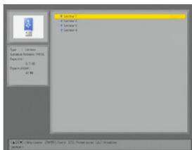
Affichage arborescent
