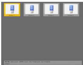
Affichage d'icônes
