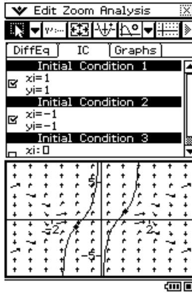
Editeur de conditions initiales (onglet [IC])
