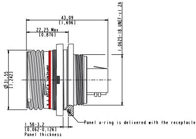
RJF TV 7 1 X F312 Receptacle CAT5e
