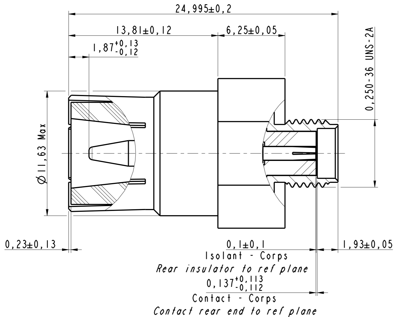
COUPE A-A SECTION A-A
