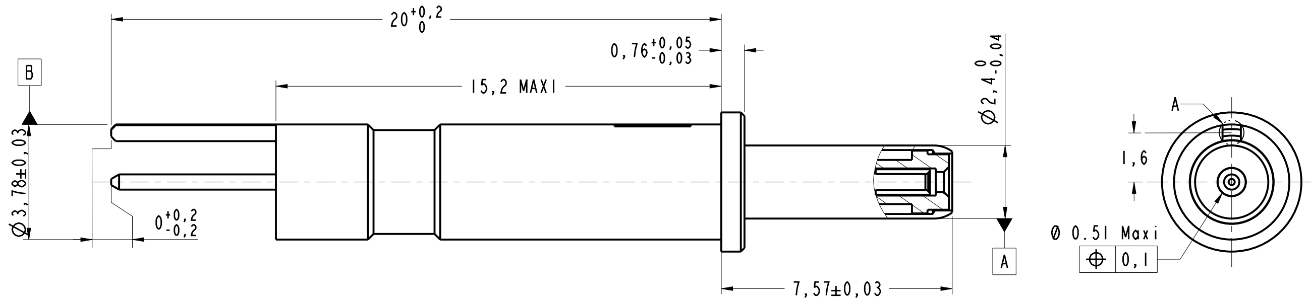
COUPE A-A
